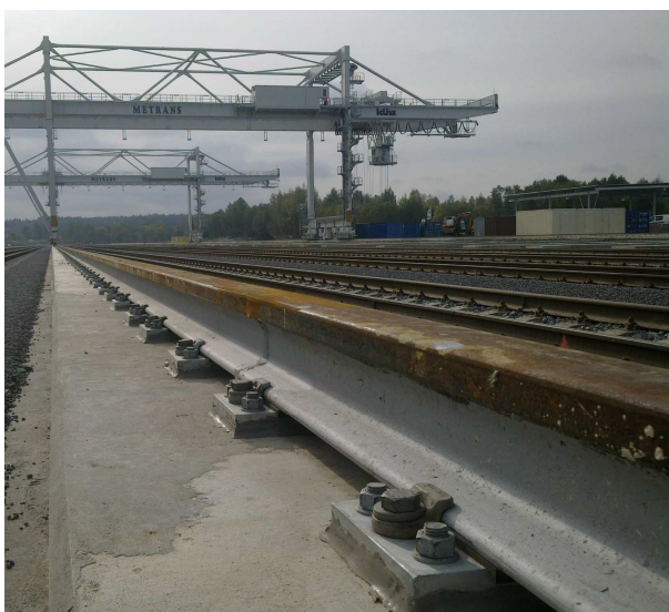
▲ kotvení podkladnic
