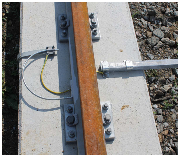
▲ provedení uzemnění jeřábové dráhy
